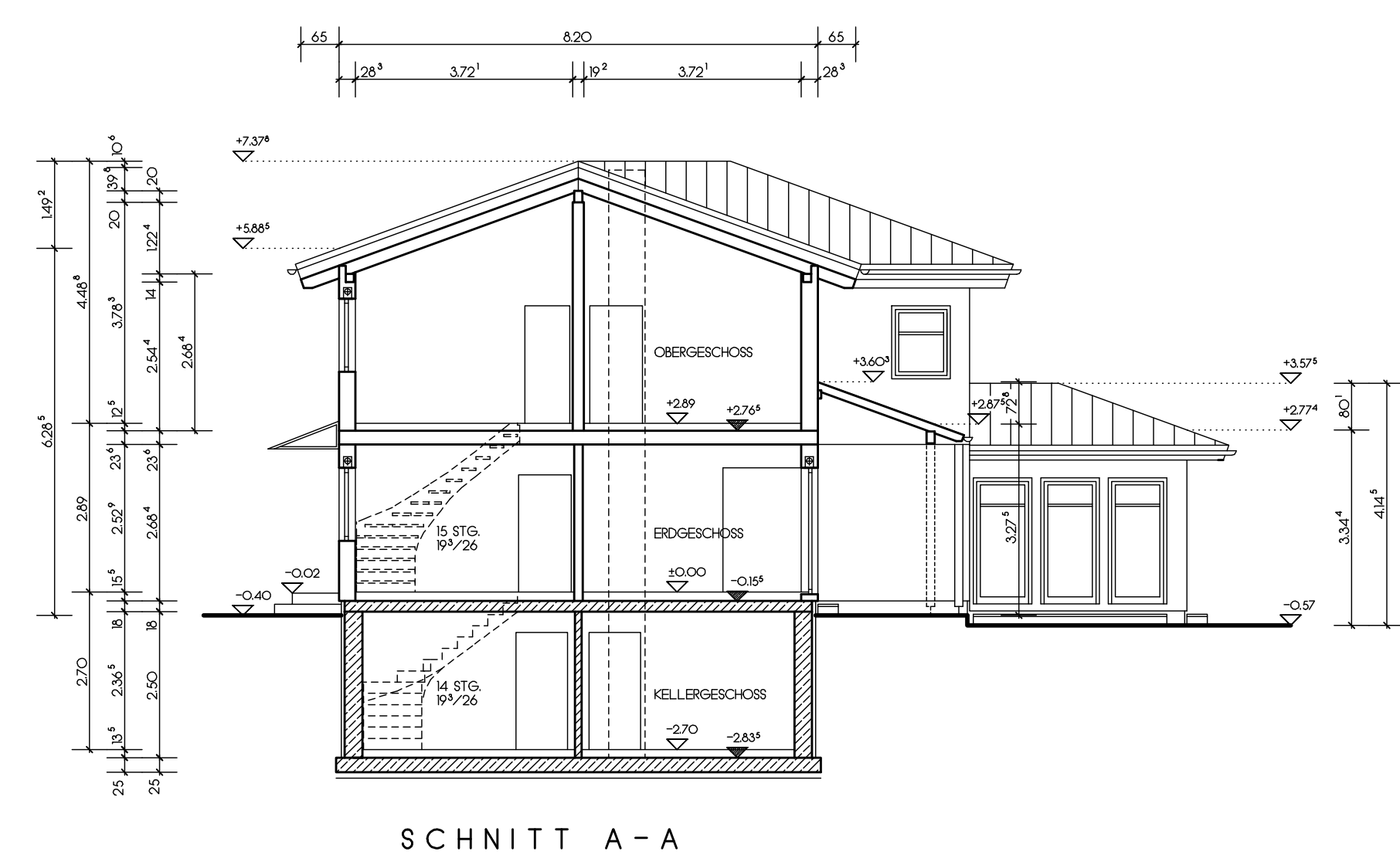
SCHNITT A-A
